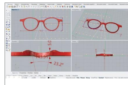
Programas
